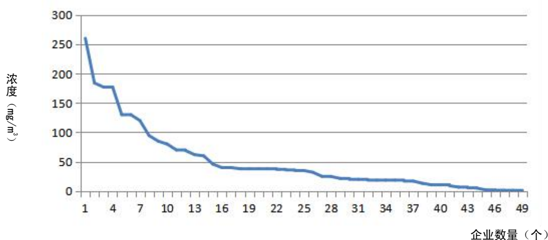
图 5-18 燃气炉氮氧化物排放浓度统计 ( \text{mg}/\text{m}^3 )
