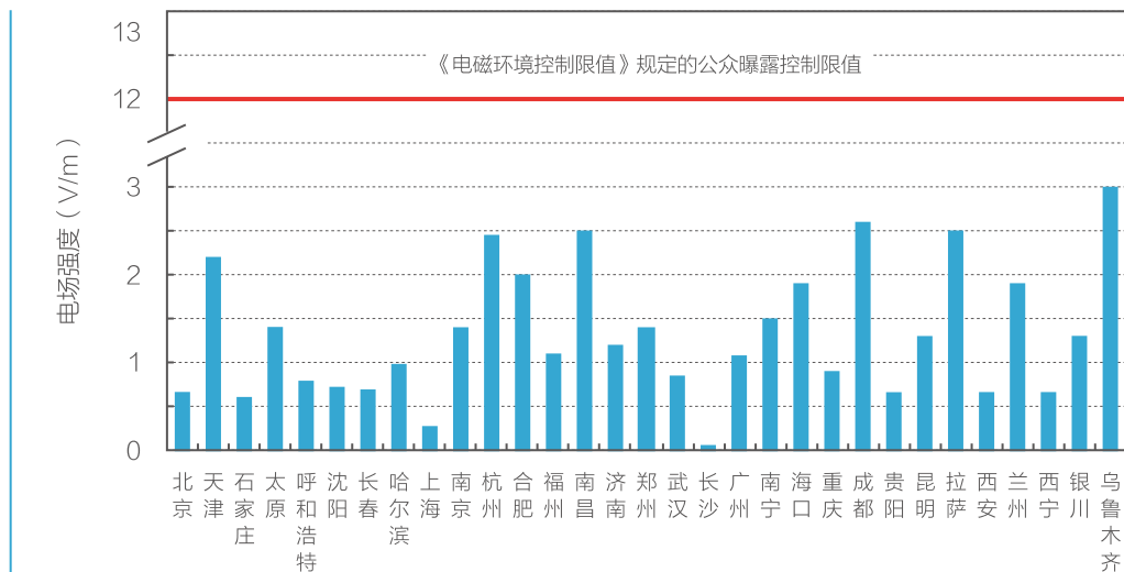
图 3.5-2 环境电磁辐射水平
