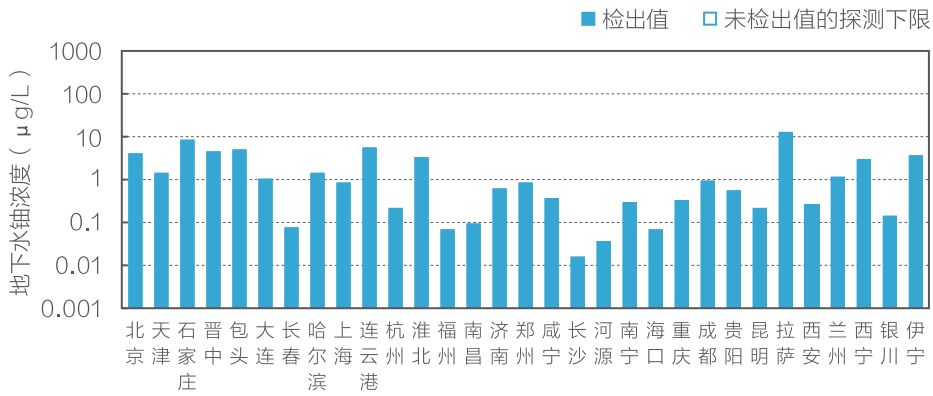
图 3.3.3-4 地下水中铀浓度
