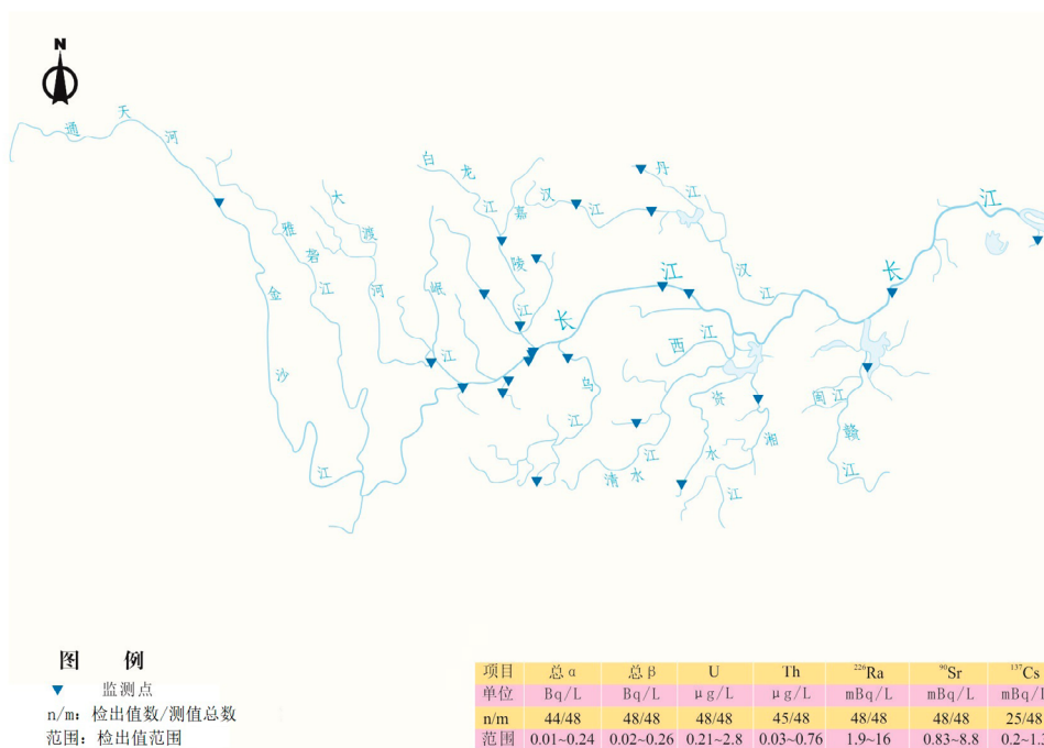
图 3.3.1-1 长江流域布点和监测结果示意图
