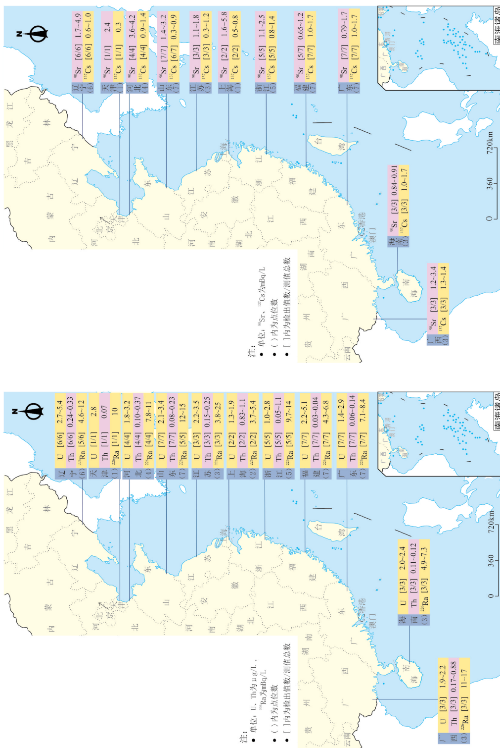
图 3.3.5-1 近岸海域海水监测结果
