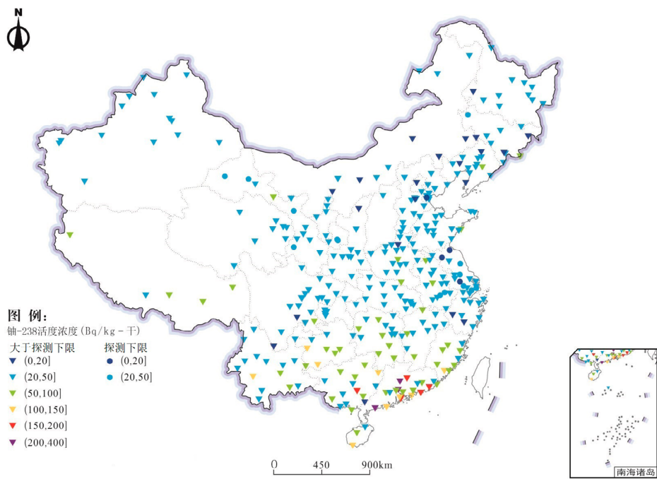
图 3.4-1 土壤中轴-238活度浓度分布示意图
