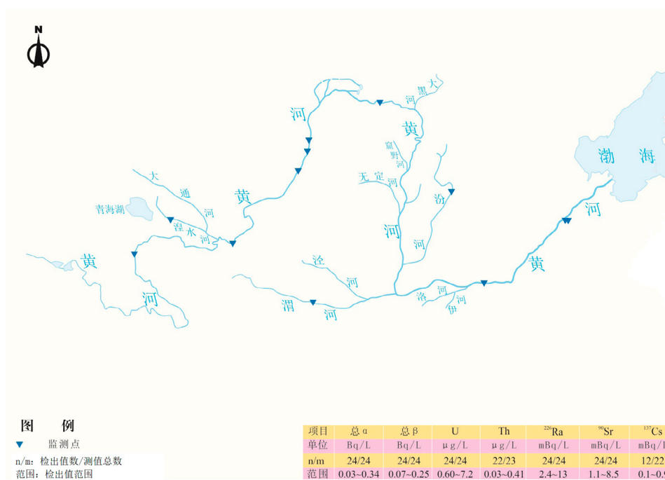
图 3.3.1-2 黄河流域布点和监测结果示意图
