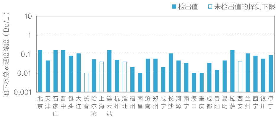
图 3.3.3-2 地下水中总 \alpha 活度浓度
