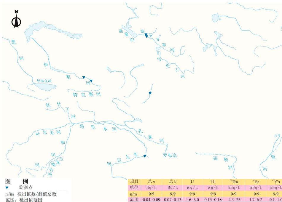
图 3.3.1-9 西北诸河布点和监测结果示意图
