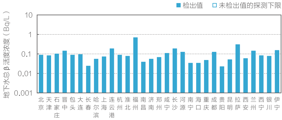
图 3.3.3-3 地下水中总β活度浓度
