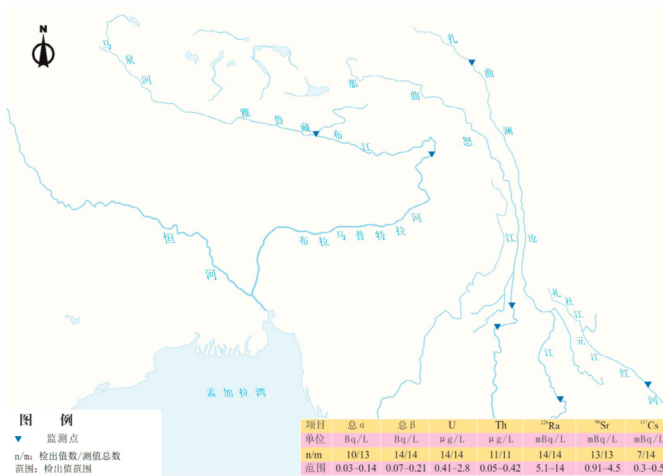
图 3.3.1-10 西南诸河布点和监测结果示意图
