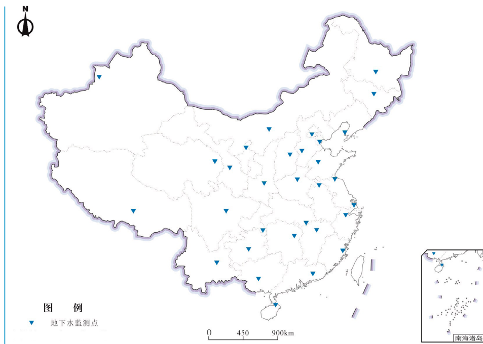
图 3.3.3-1 地下水布点示意图
